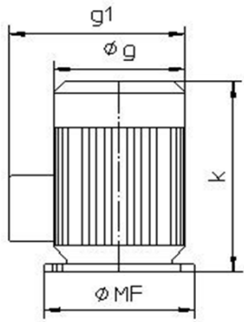
Bauform V1
