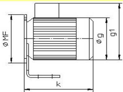
Bauform B5
