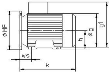
Bauform B35
